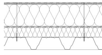
Stahltrapezprofildach, Modernisierung durch Aufdopplung
