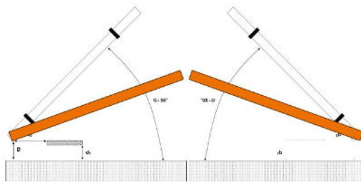
PV-Anordnung, PV-Neigungswinkel und Brennerpositionierung in Anlehnung an CLC/TR 50670
